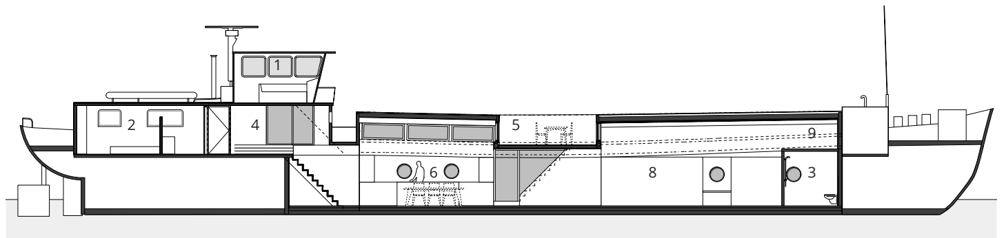
DOORSNEDE
