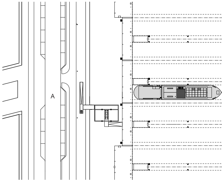
SITUATIE
