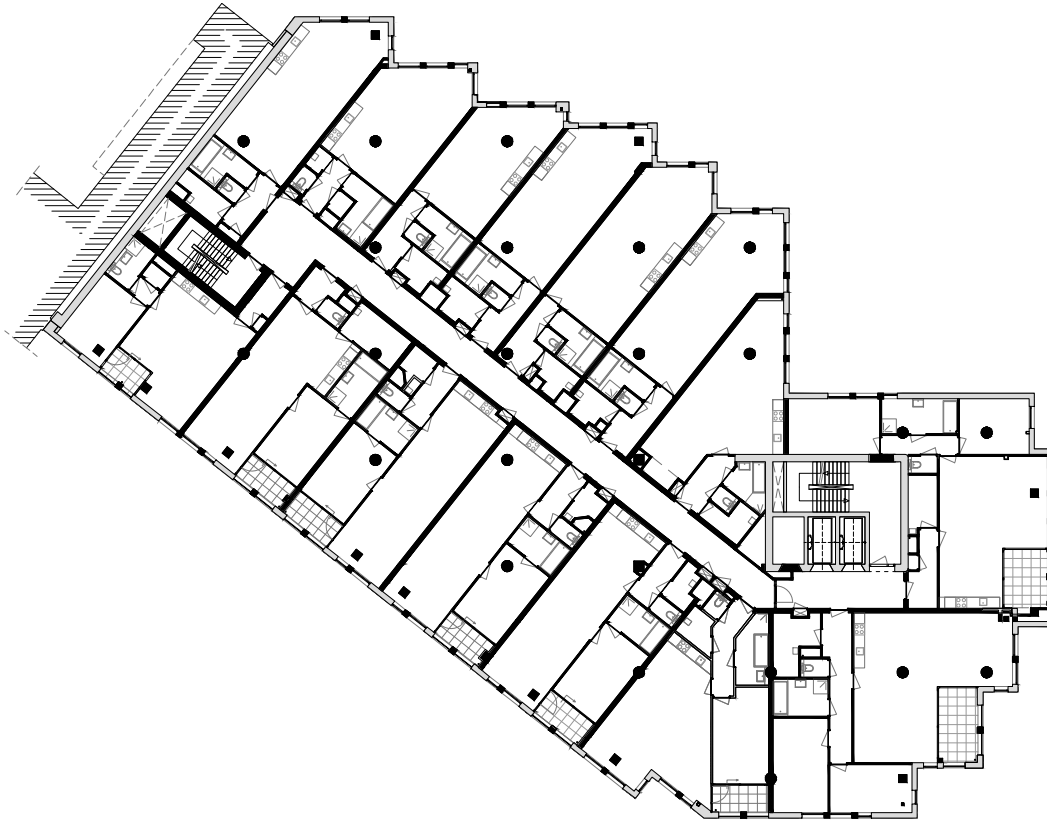
eerste verdieping
