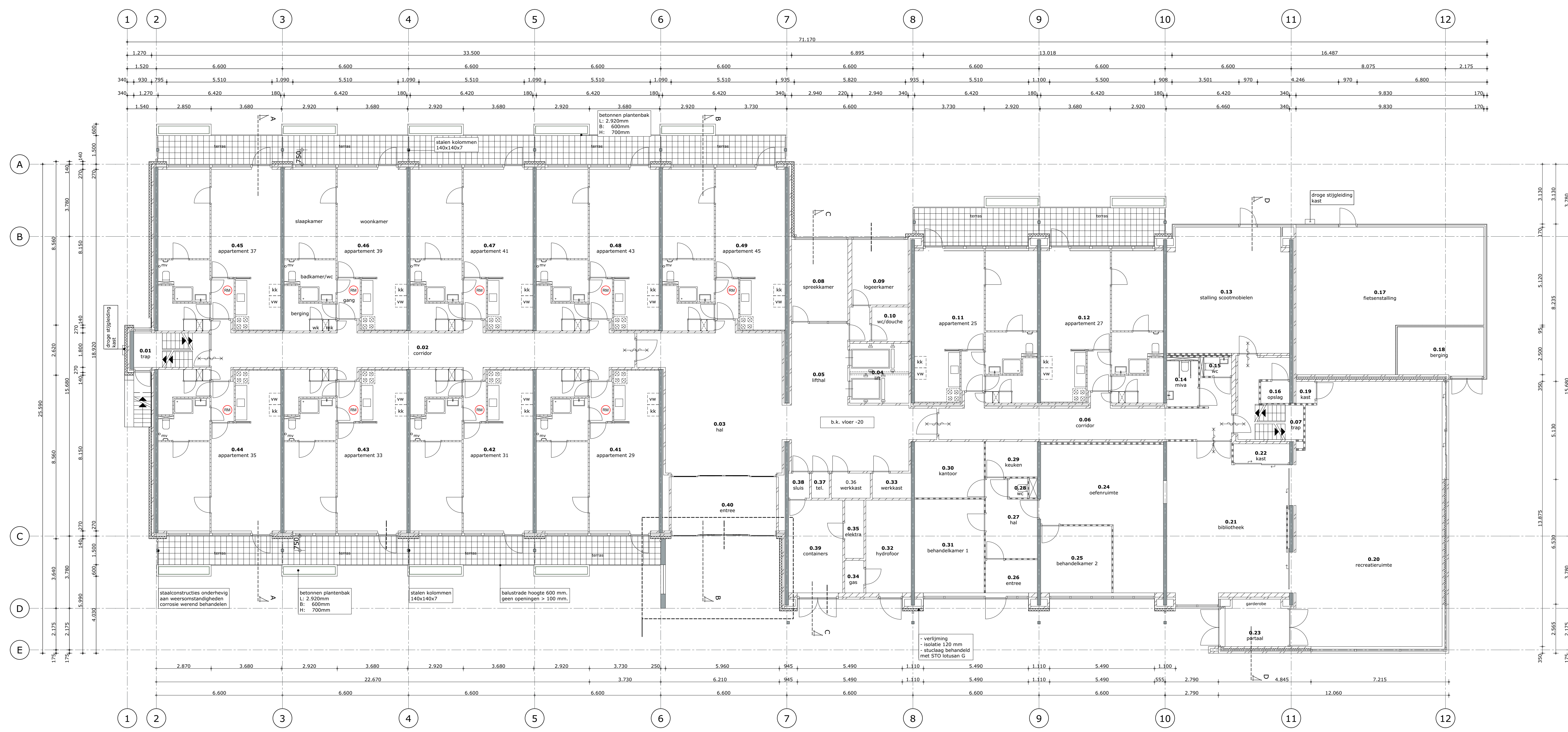
BEGANE GROND
